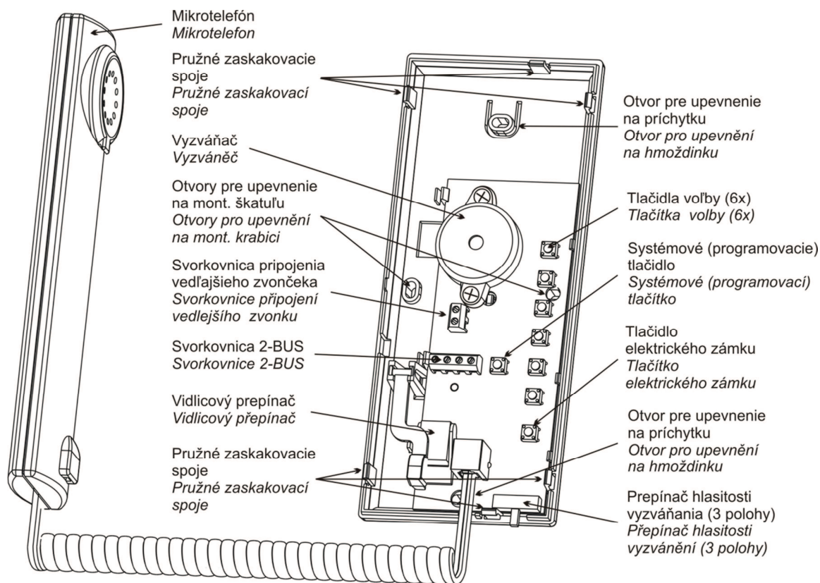
Obr. 2 Montážne, nastavovacie a ovládacie prvky DT prístupné po odobratí vrchného krytu Montážní, nastavovací a ovládací prvky DT přístupné po sejmутí vrchního krytu
